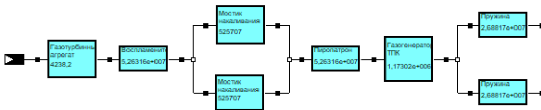
Рисунок 3. Фрагмент блок-схемы надёжности зенитной управляемой ракеты
