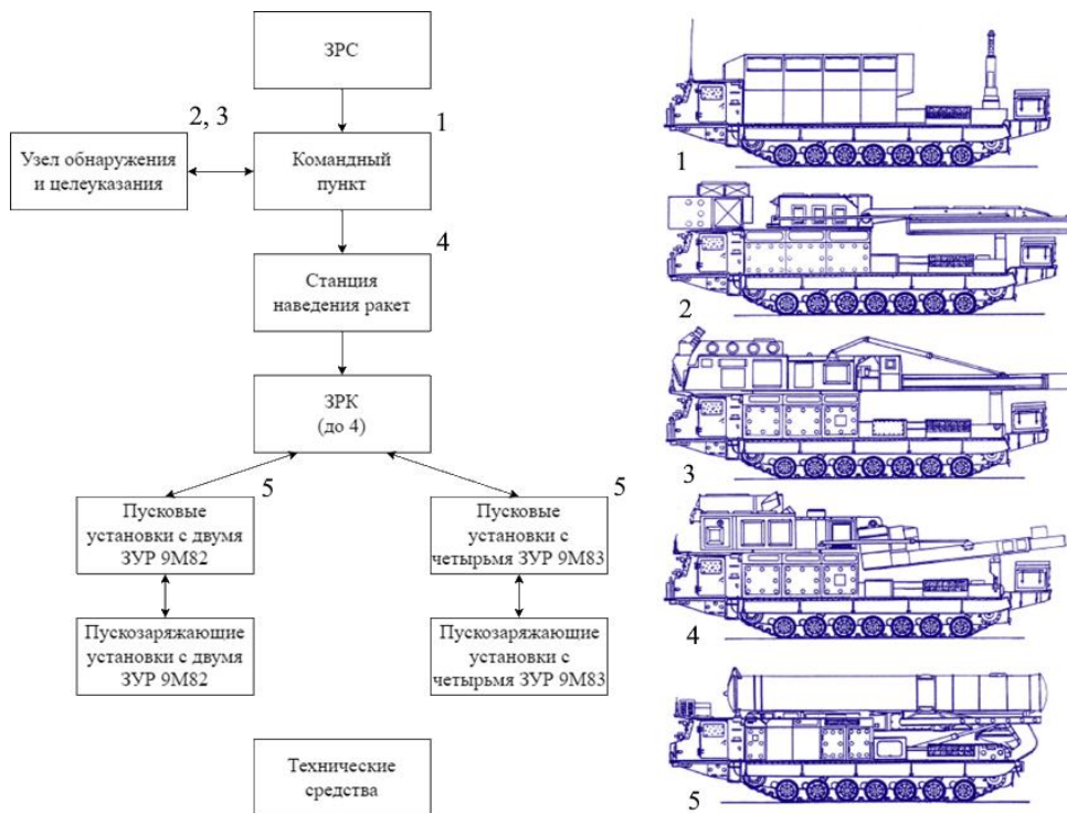
Рисунок 1. Структура ЗРС С-300В
