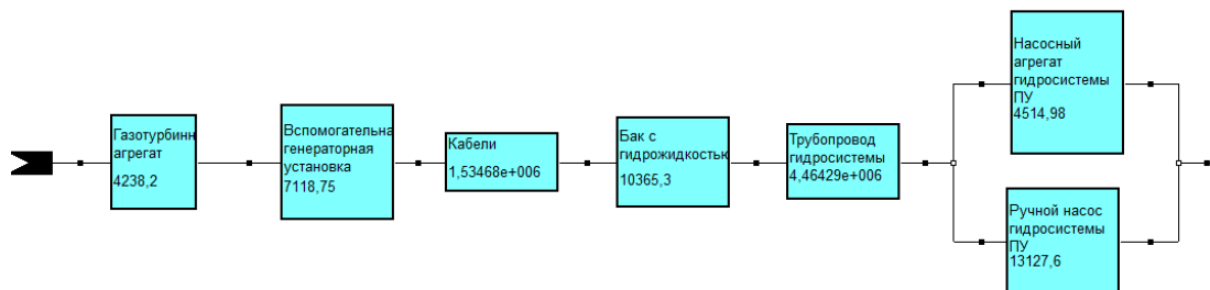
Рисунок 2. Фрагмент блок-схемы надёжности пусковой установки
