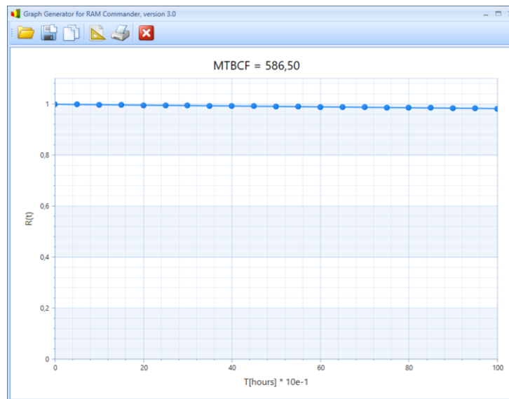
Рисунок 7. Анализ МТВСФ и R(t) блок-схемы ЗРК
